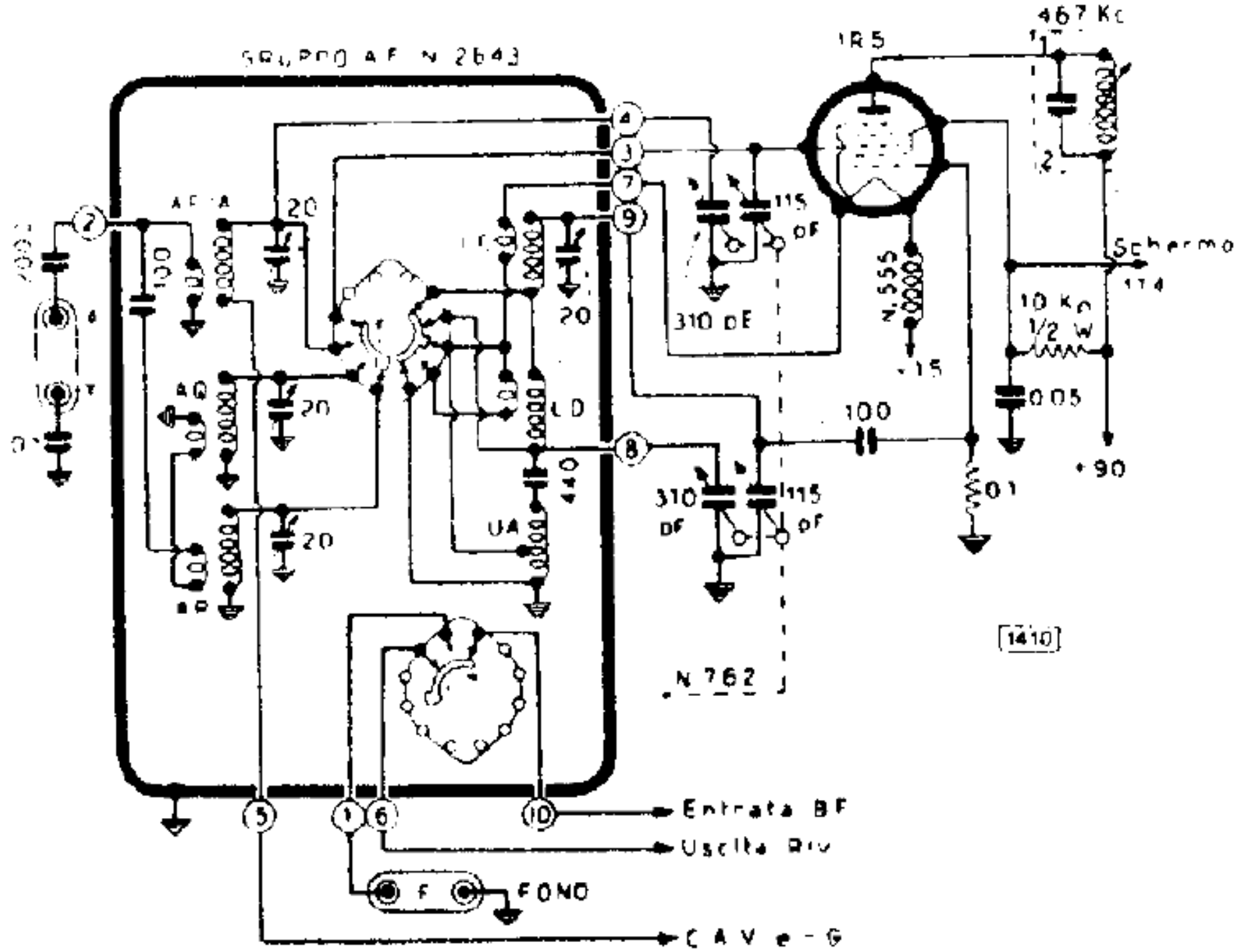
Commutatore visto di dietro nella pos onde più corte
